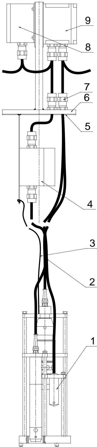
1 - блок датчиков; 2 - кабель (3 шт.); 3 - металлический тросик; 4 – защитная коробка капилляра; 5 - паранитовая прокладка; 6 – фланец; 7 – кабельные вводы; 8 – контроллер КИ; 9 – клемная коробка.
