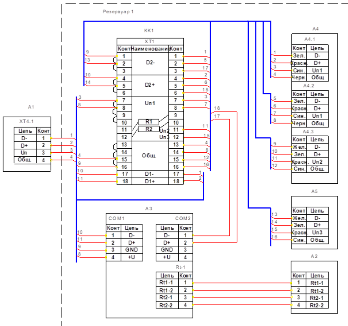
Рисунок 6 Контроллер КИ
